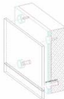
KOTWIENIE W FUDZE POZIOMEJ - KOTWY NOŚNE RURIOWE
